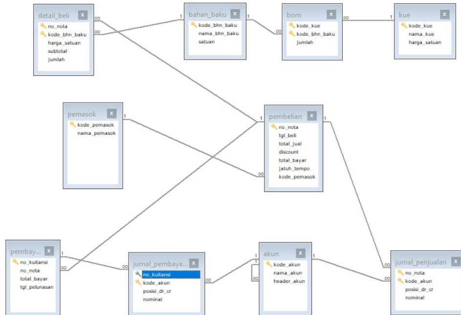
Gambar 1. Kueri DLL
